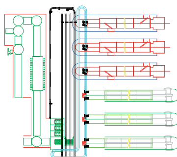
Layout-Beispiel: OE-Spinnerei Layout example: OE-spinning plant
