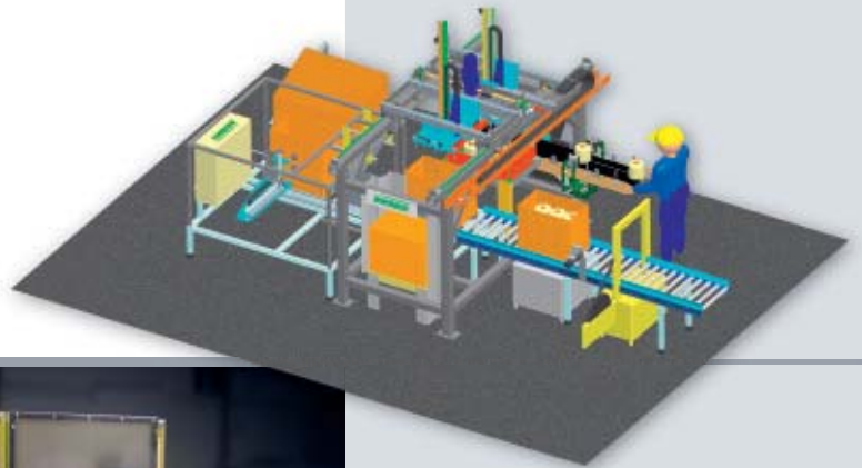
Kartonverpackungsmaschine Box packing machine
