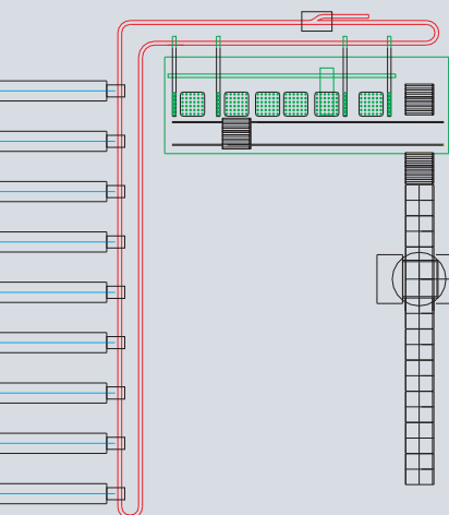
Layout-Beispiel: Ringspinnerei Layout example: Ring spinning plant
